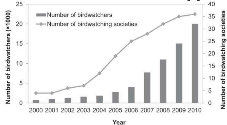
中国におけるバードウォッチングをする人と バードウォッチング協会の数の推移 [6]
